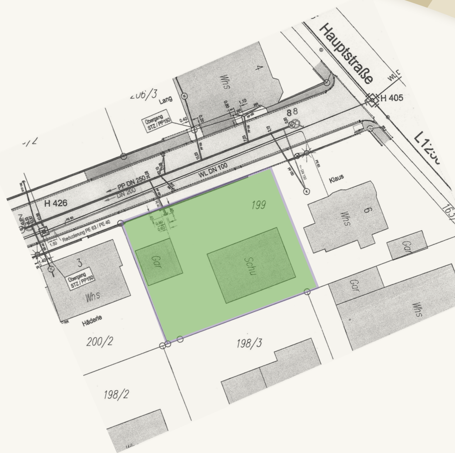
Erschließungsplan - Wasser -
