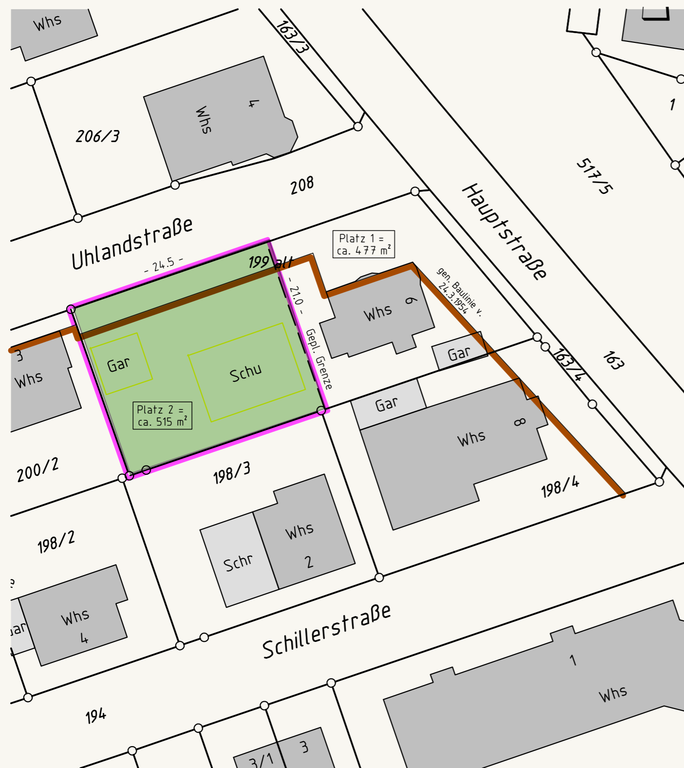
Lageplan
